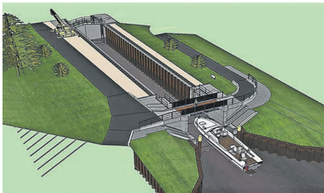
Der Entwurf gibt einen Eindruck von der Größe des Bauprojekts: Die Schleuse wird ganze 41,5 Meter lang und sechs Meter breit.
